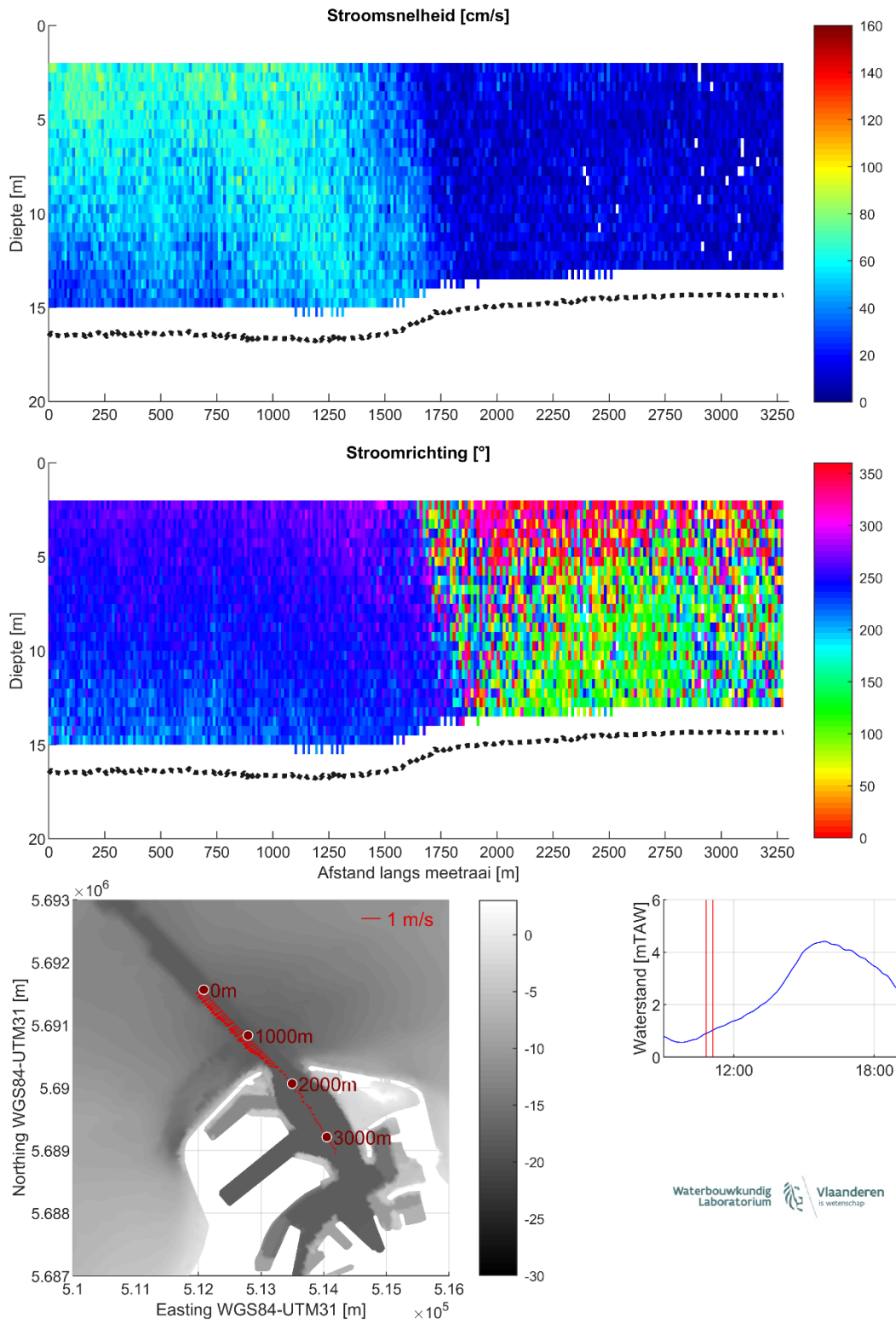
Figuur 9 – Stroomgegevens 18/08/2023 raai 4: snelheidsgrootte (top), -richting (midden) en diepte-gemiddelde vectoren (onder)
