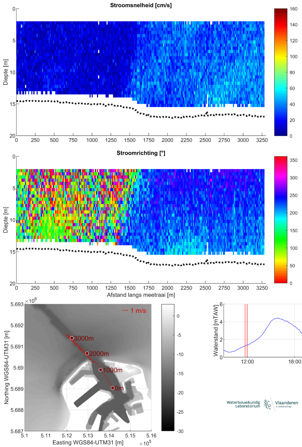
Figuur 12 – Stroomgegevens 18/08/2023 raai 7: snelheids grootte (top), -richting (midden) en diepte-gemiddelde vectoren (onder)
