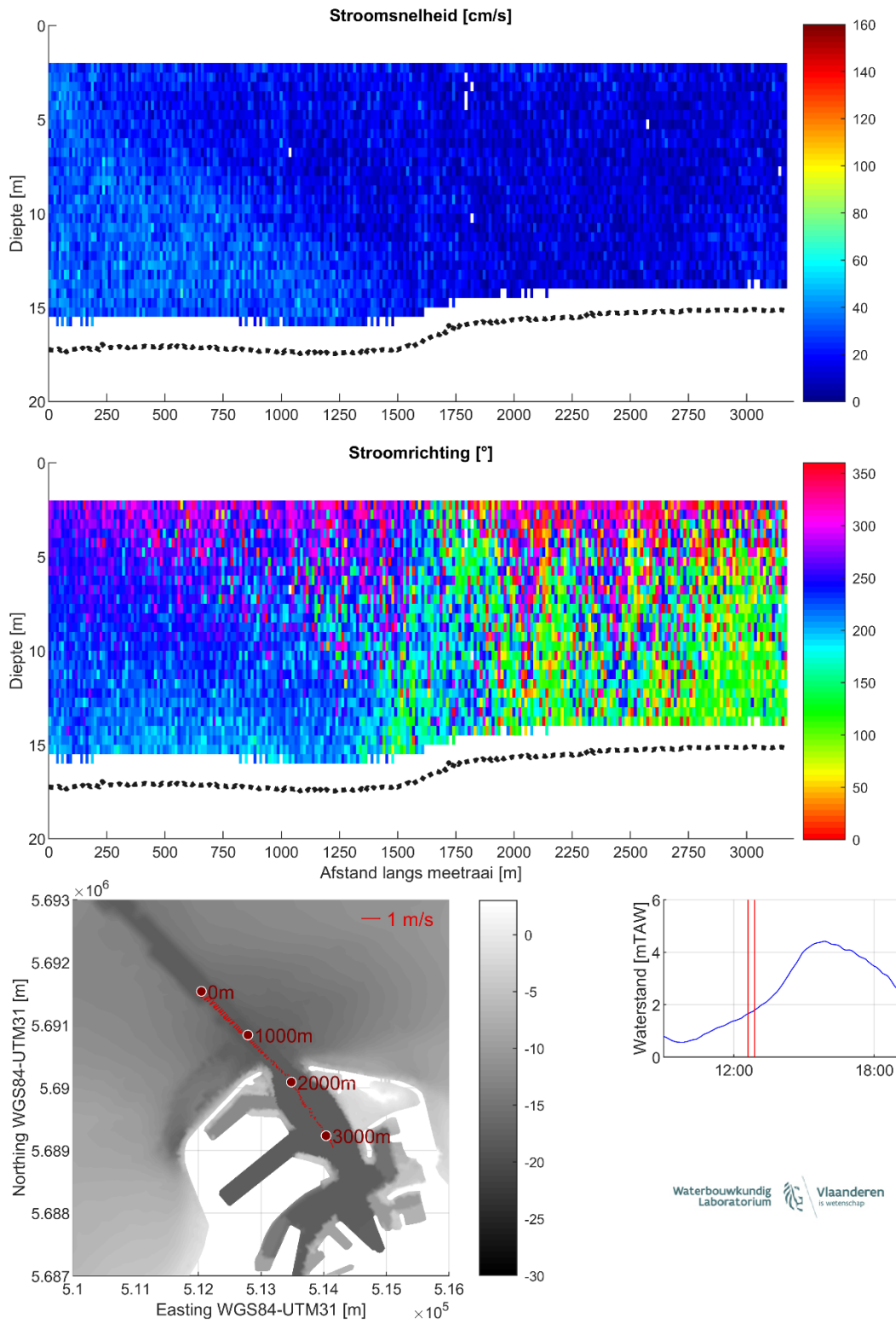
Figuur 15 – Stroomgegevens 18/08/2023 raai 10: snelheids grootte (top), -richting (midden) en diepte-gemiddelde vectoren (onder)
