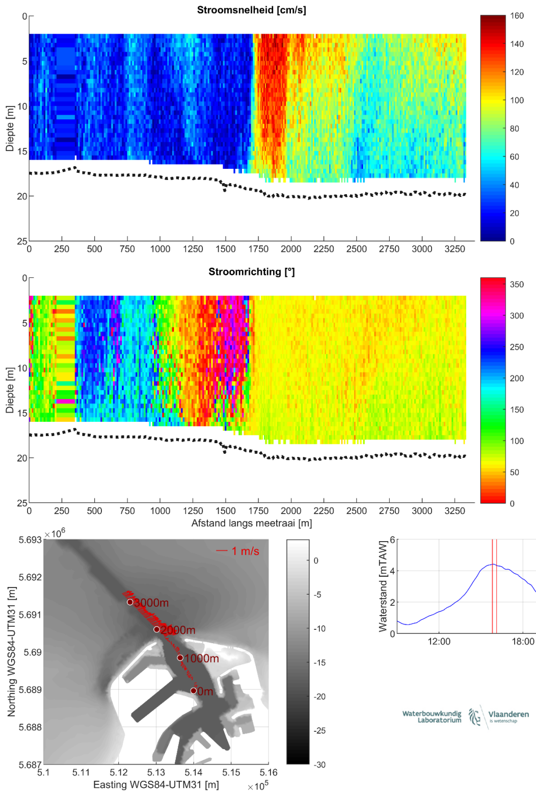
Figuur 26 – Stroomgegevens 18/08/2023 raai 21: snelheids grootte (top), -richting (midden) en diepte-gemiddelde vectoren (onder)
