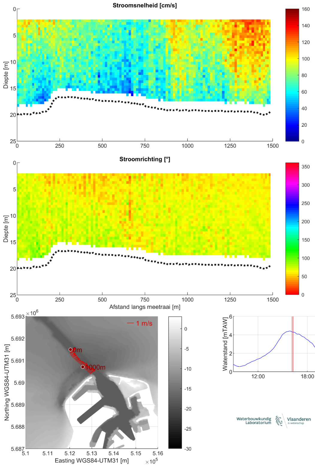
Figuur 27 – Stroomgegevens 18/08/2023 raai 22: snelheids grootte (top), -richting (midden) en diepte-gemiddelde vectoren (onder)
