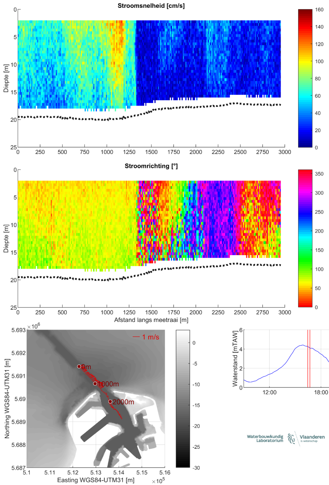
Figuur 29 – Stroomgegevens 18/08/2023 raai 24: snelheids grootte (top), -richting (midden) en diepte-gemiddelde vectoren (onder)
