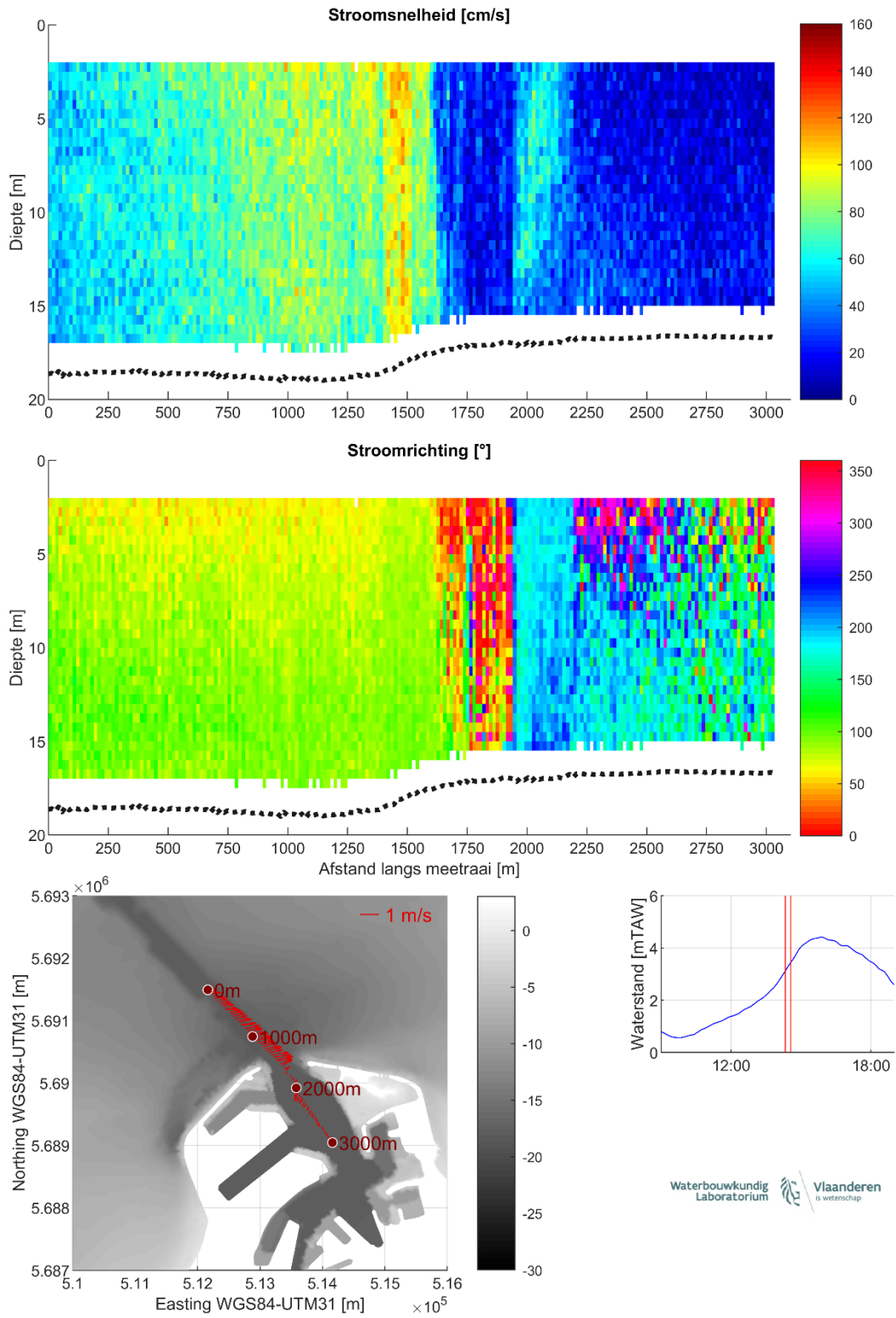
Figuur 21 – Stroomgegevens 18/08/2023 raai 16: snelheids grootte (top), -richting (midden) en diepte-gemiddelde vectoren (onder)
