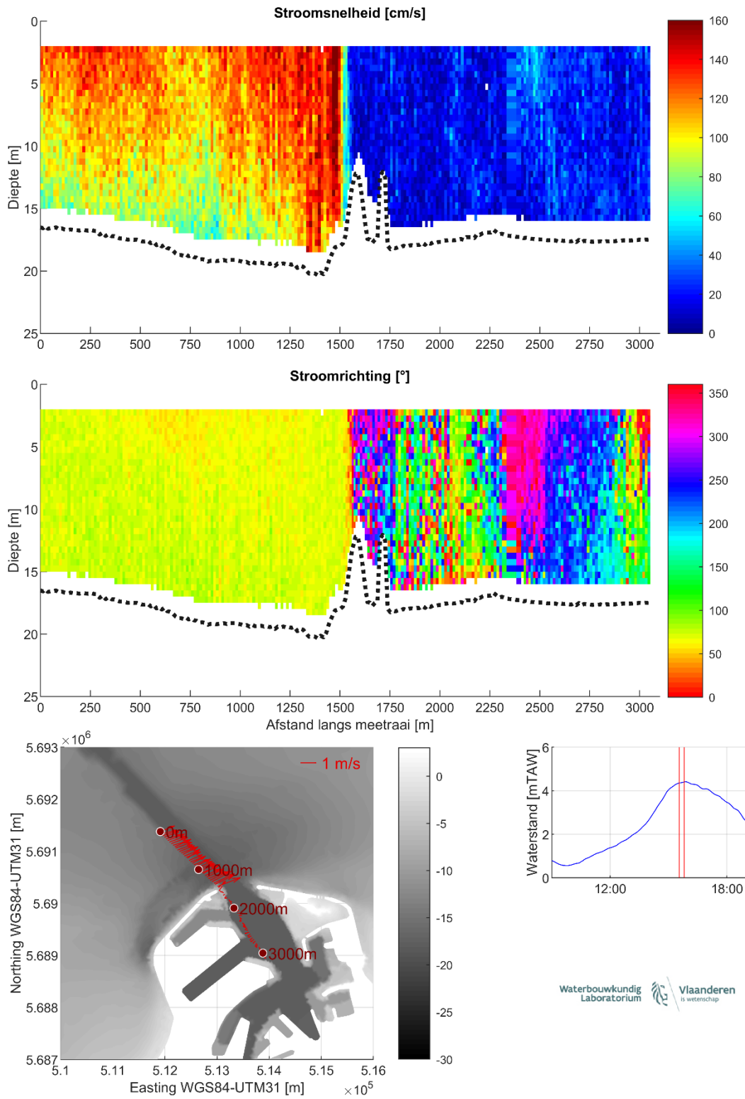
Figuur 25 – Stroomgegevens 18/08/2023 raai 20: snelheidsgrootte (top), -richting (midden) en diepte-gemiddelde vectoren (onder)
