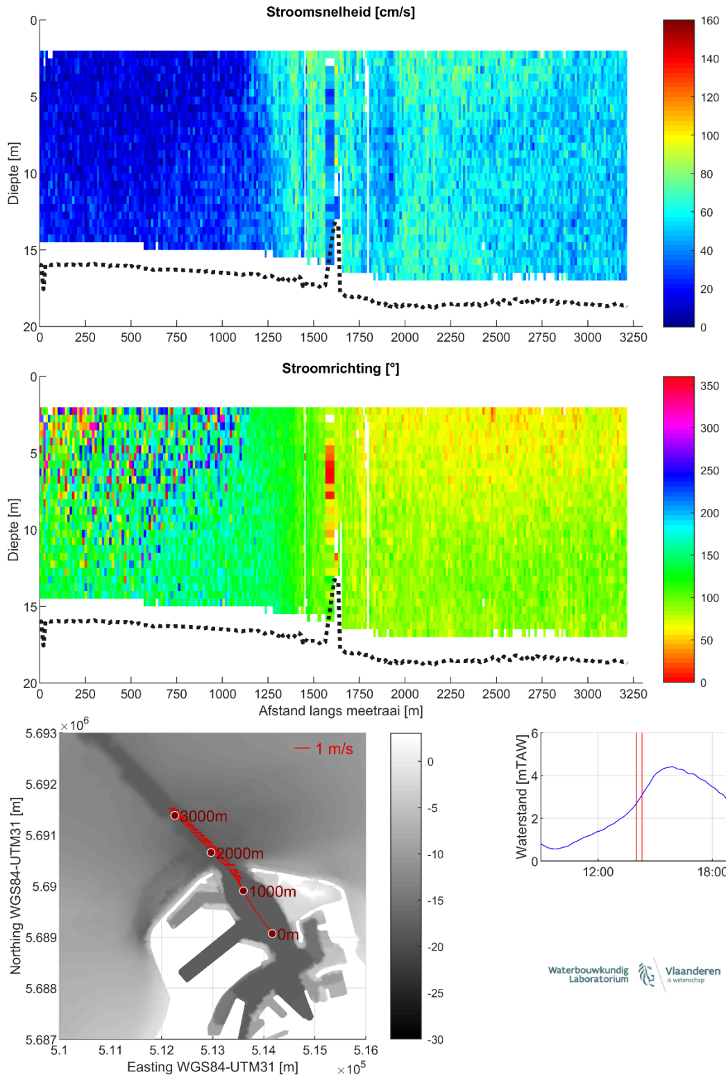
Figuur 20 – Stroomgegevens 18/08/2023 raai 15: snelheids grootte (top), -richting (midden) en diepte-gemiddelde vectoren (onder)
