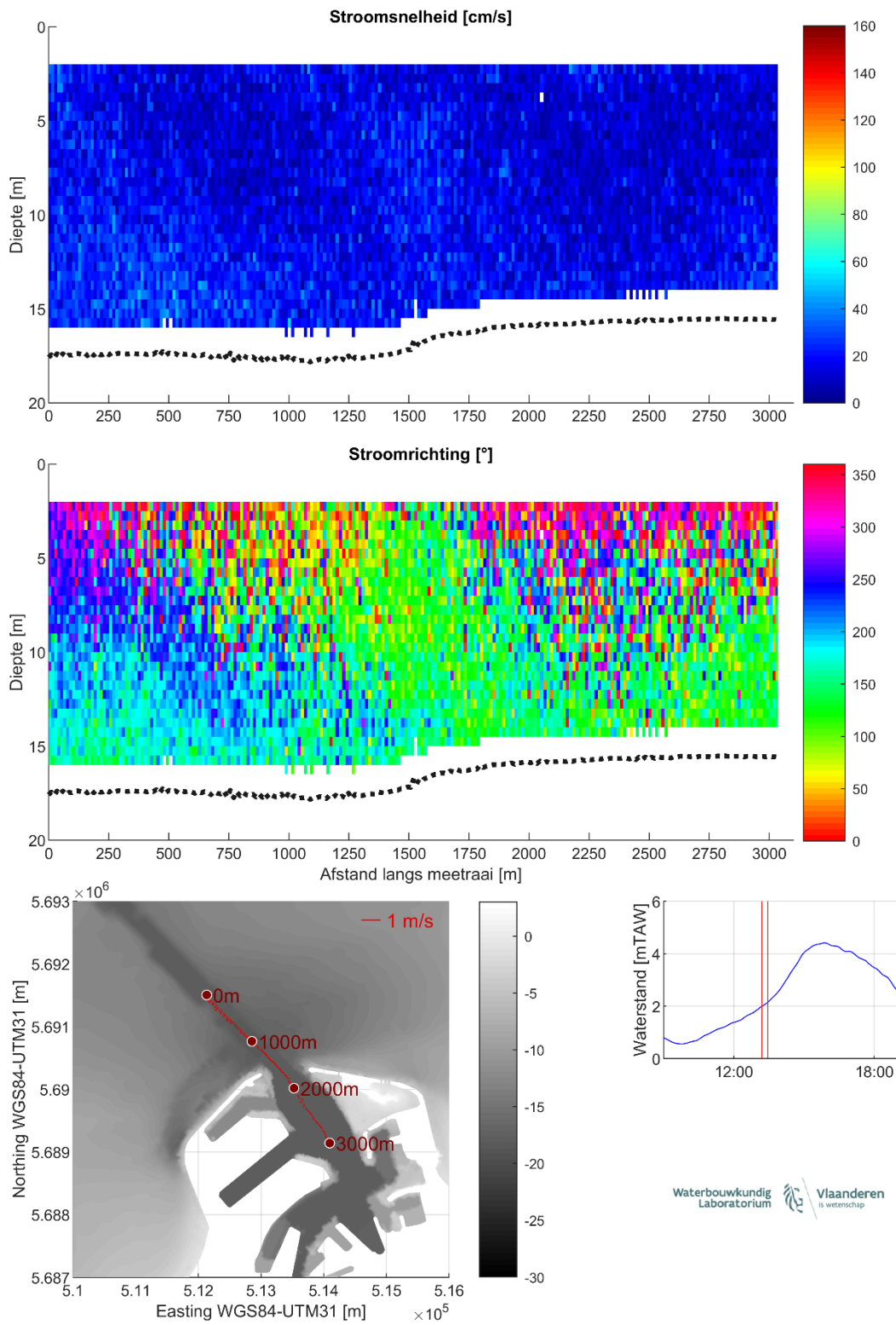
Figuur 17 – Stroomgegevens 18/08/2023 raai 12: snelheids grootte (top), -richting (midden) en diepte-gemiddelde vectoren (onder)
