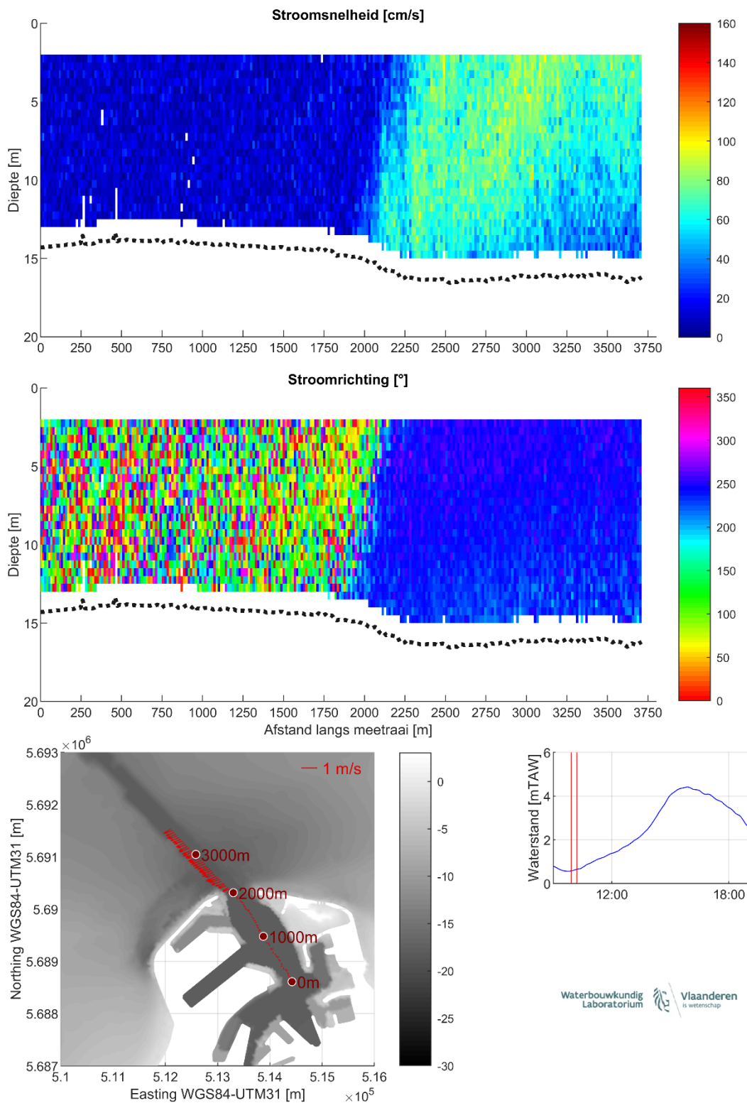
Figuur 6 – Stroomgegevens 18/08/2023 raai 1: snelheidsgrootte (top), -richting (midden) en diepte-gemiddelde vectoren (onder)
