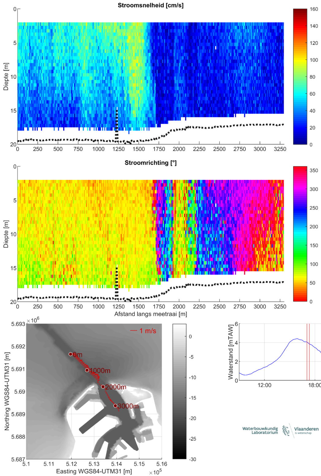
Figuur 31 – Stroomgegevens 18/08/2023 raai 26: snelheids grootte (top), -richting (midden) en diepte-gemiddelde vectoren (onder)
