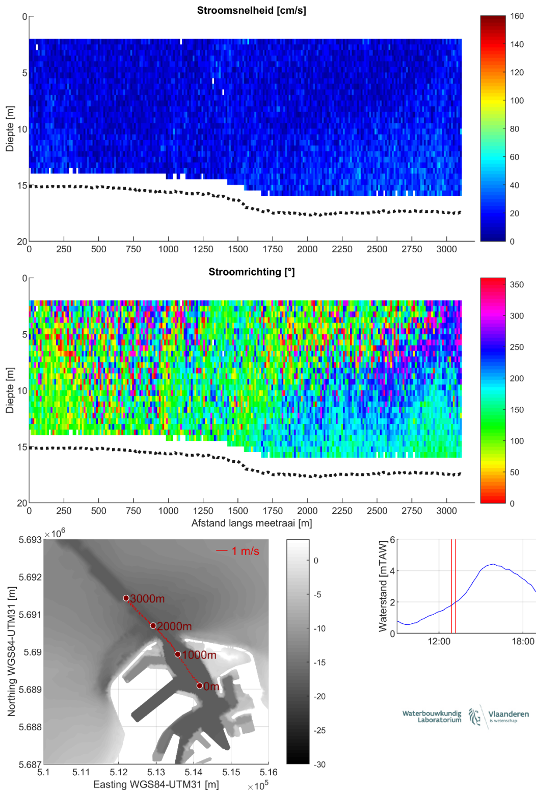
Figuur 16 – Stroomgegevens 18/08/2023 raai 11: snelheids grootte (top), -richting (midden) en diepte-gemiddelde vectoren (onder)
