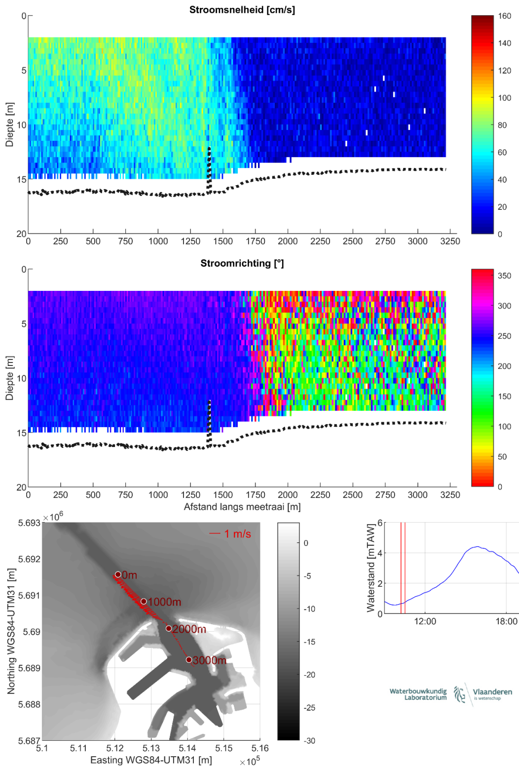
Figuur 7 – Stroomgegevens 18/08/2023 raai 2: snelheids grootte (top), -richting (midden) en diepte-gemiddelde vectoren (onder)
