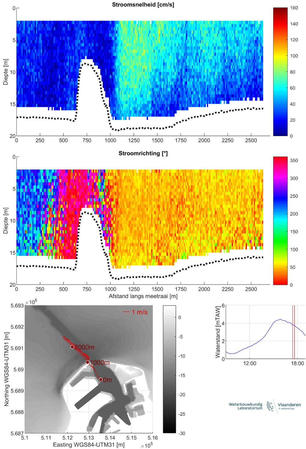
Figuur 32 – Stroomgegevens 18/08/2023 raai 27: snelheids grootte (top), -richting (midden) en diepte-gemiddelde vectoren (onder)
