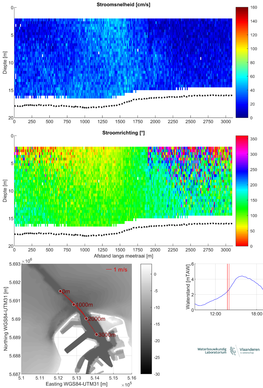
Figuur 19 – Stroomgegevens 18/08/2023 raai 14: snelheids grootte (top), -richting (midden) en diepte-gemiddelde vectoren (onder)
