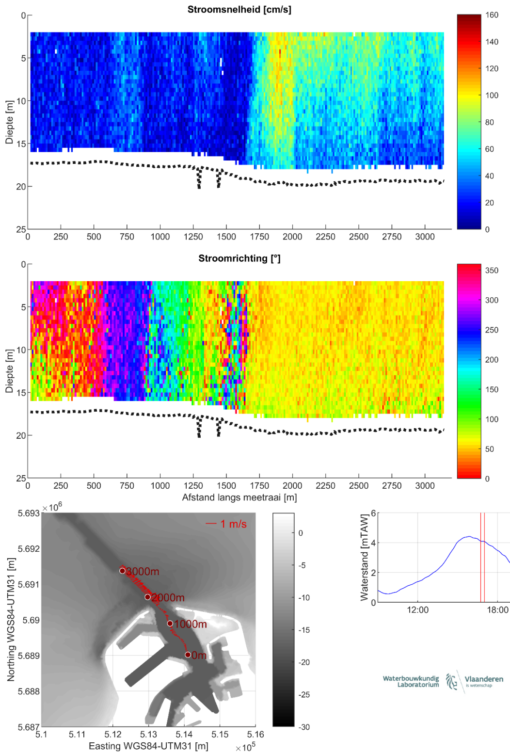
Figuur 30 – Stroomgegevens 18/08/2023 raai 25: snelheids grootte (top), -richting (midden) en diepte-gemiddelde vectoren (onder)
