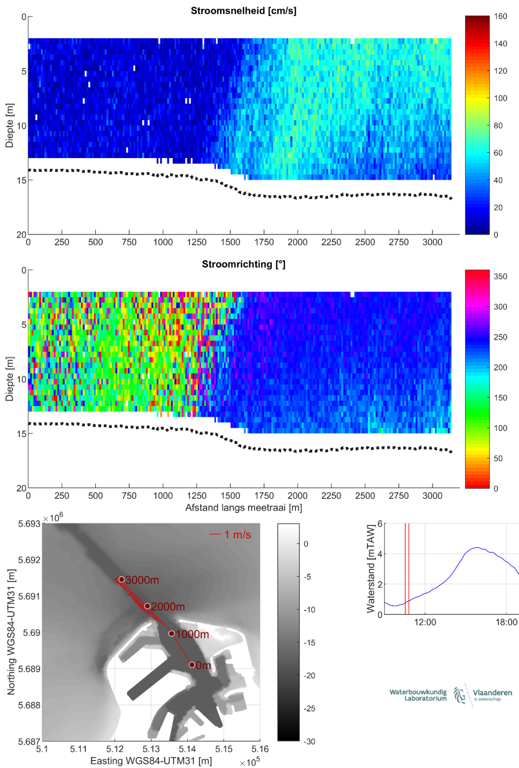
Figuur 8 – Stroomgegevens 18/08/2023 raai 3: snelheidsgrootte (top), -richting (midden) en diepte-gemiddelde vectoren (onder)
