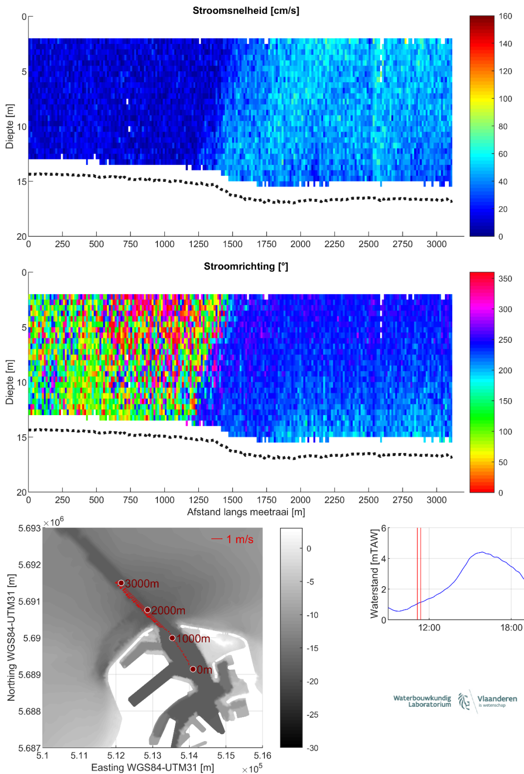
Figuur 10 – Stroomgegevens 18/08/2023 raai 5: snelheids grootte (top), -richting (midden) en diepte-gemiddelde vectoren (onder)
