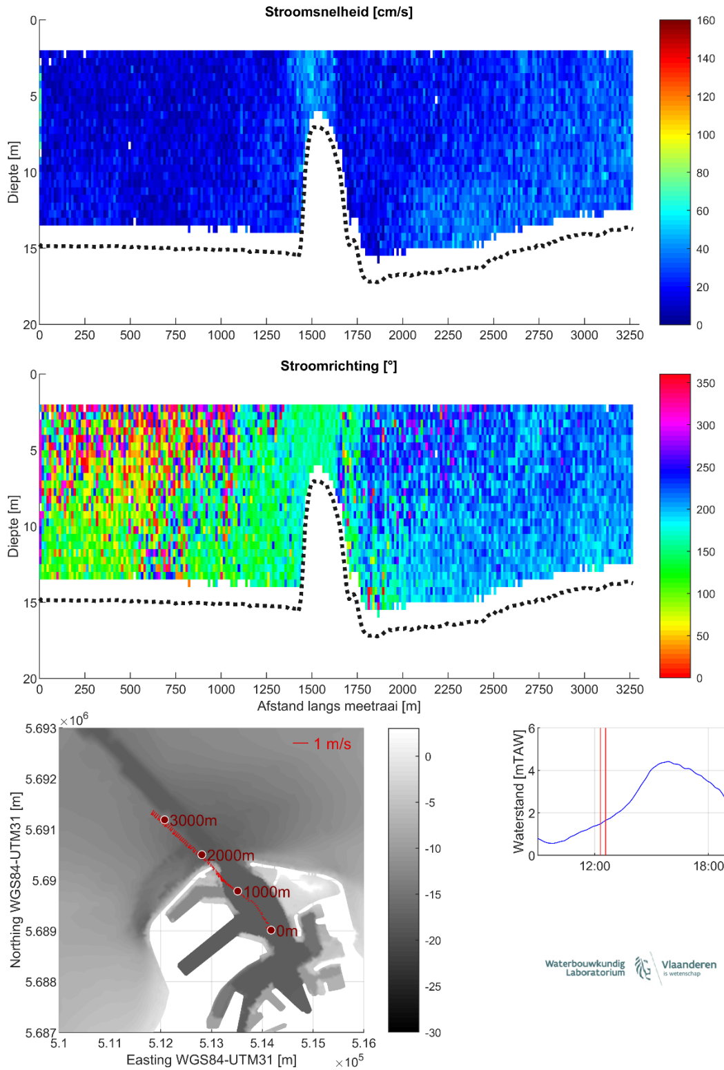
Figuur 14 – Stroomgegevens 18/08/2023 raai 9: snelheids grootte (top), -richting (midden) en diepte-gemiddelde vectoren (onder)
