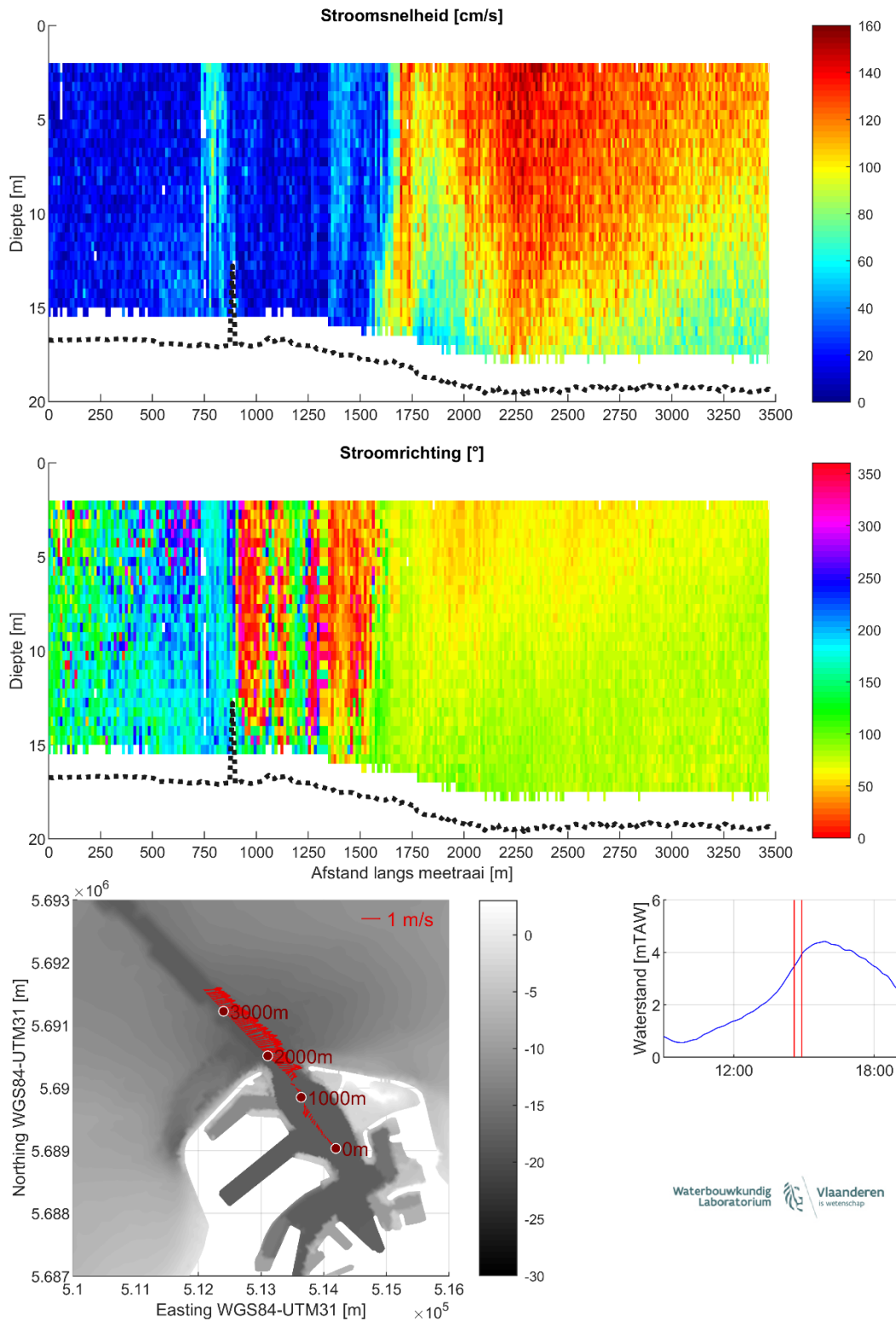
Figuur 22 – Stroomgegevens 18/08/2023 raai 17: snelheids grootte (top), -richting (midden) en diepte-gemiddelde vectoren (onder)
