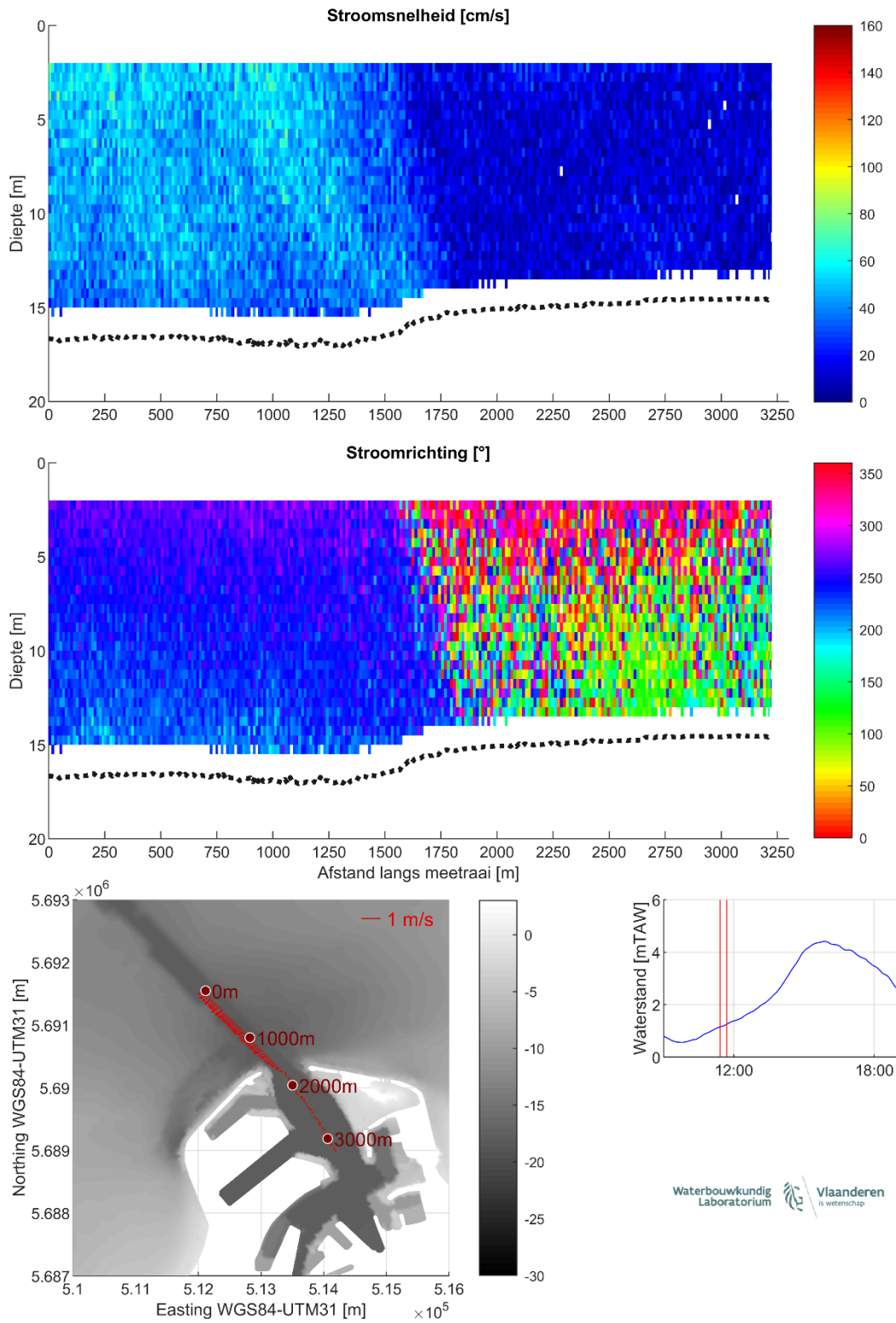
Figuur 11 – Stroomgegevens 18/08/2023 raai 6: snelheidsgrootte (top), -richting (midden) en diepte-gemiddelde vectoren (onder)
