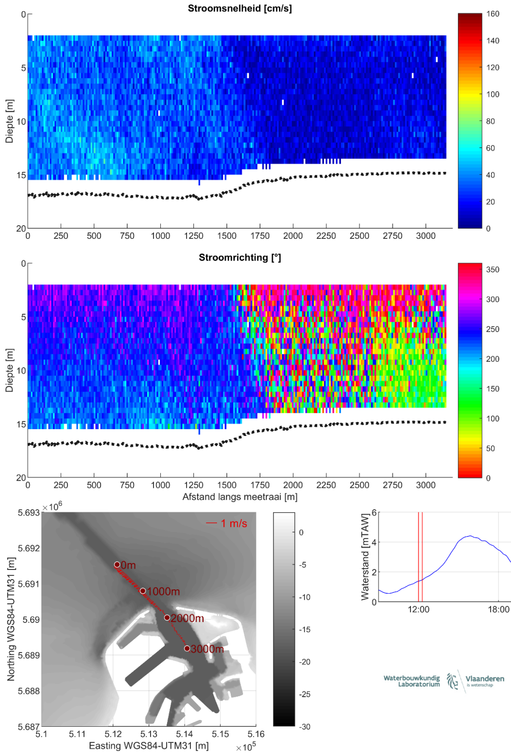
Figuur 13 – Stroomgegevens 18/08/2023 raai 8: snelheids grootte (top), -richting (midden) en diepte-gemiddelde vectoren (onder)
