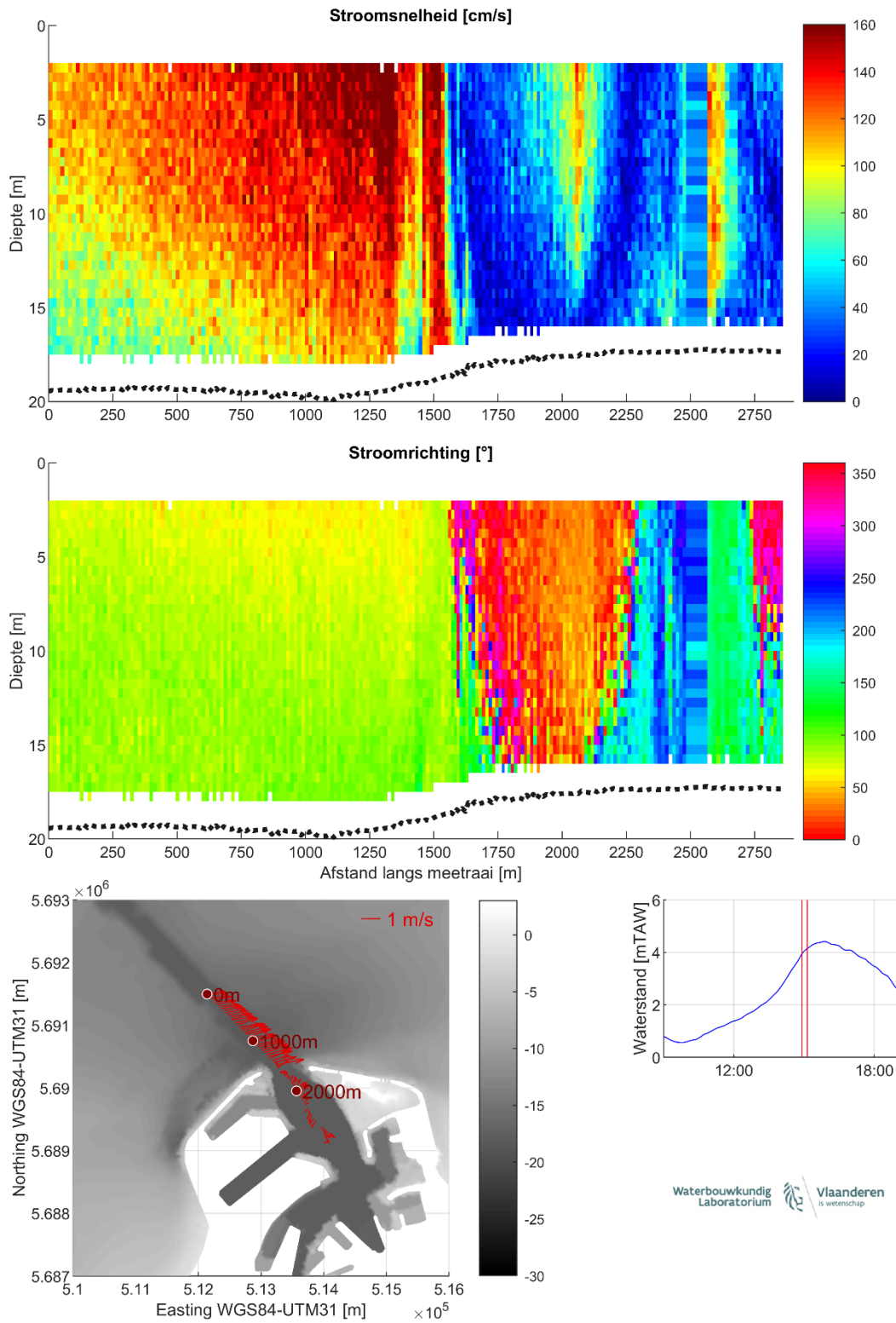
Figuur 23 – Stroomgegevens 18/08/2023 raai 18: snelheids grootte (top), -richting (midden) en diepte-gemiddelde vectoren (onder)
