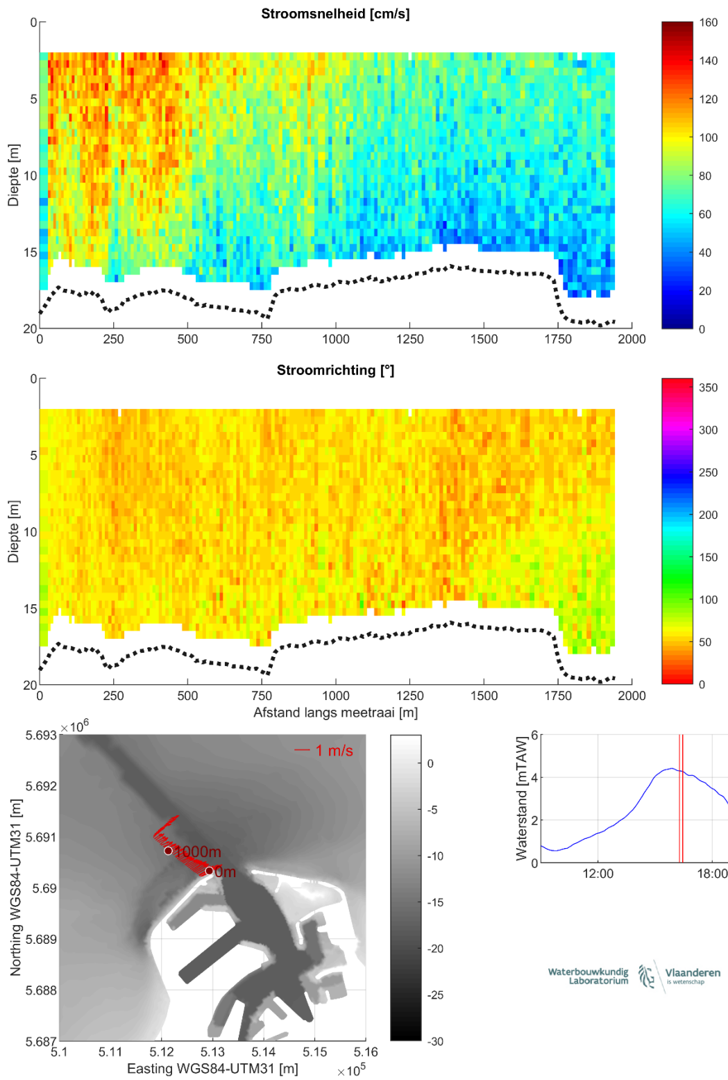
Figuur 28 – Stroomgegevens 18/08/2023 raai 23: snelheids grootte (top), -richting (midden) en diepte-gemiddelde vectoren (onder)
