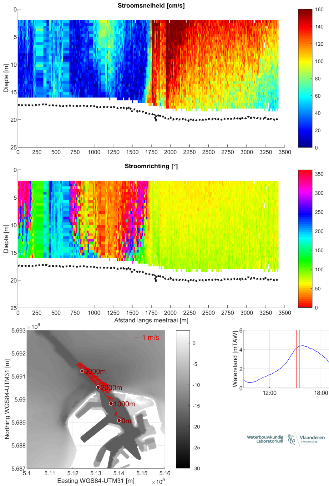
Figuur 24 – Stroomgegevens 18/08/2023 raai 19: snelheidsgrootte (top), -richting (midden) en diepte-gemiddelde vectoren (onder)
