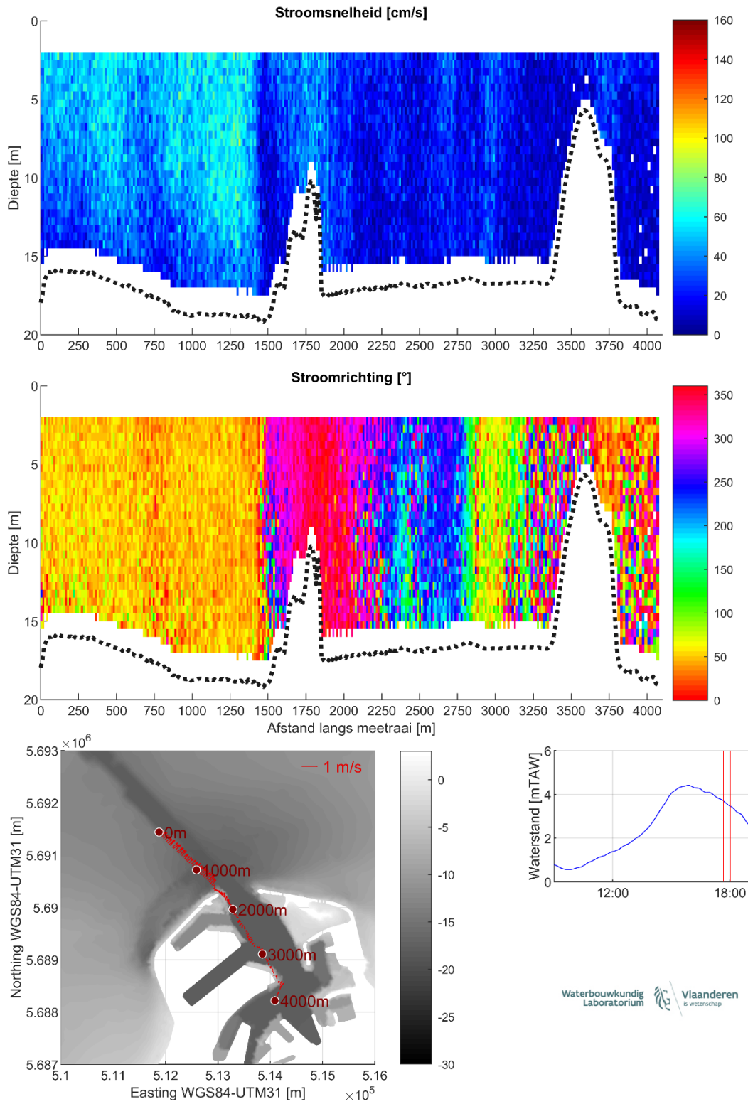
Figuur 33 – Stroomgegevens 18/08/2023 raai 28: snelheids grootte (top), -richting (midden) en diepte-gemiddelde vectoren (onder)
