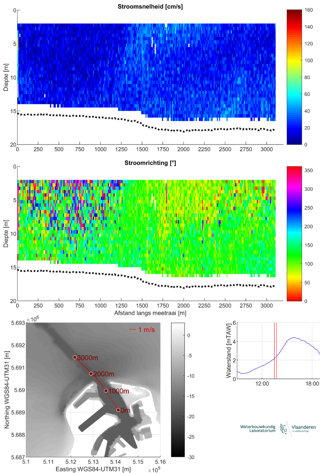
Figuur 18 – Stroomgegevens 18/08/2023 raai 13: snelheids grootte (top), -richting (midden) en diepte-gemiddelde vectoren (onder)
